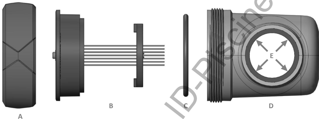
Explosionsansicht der Montage:
