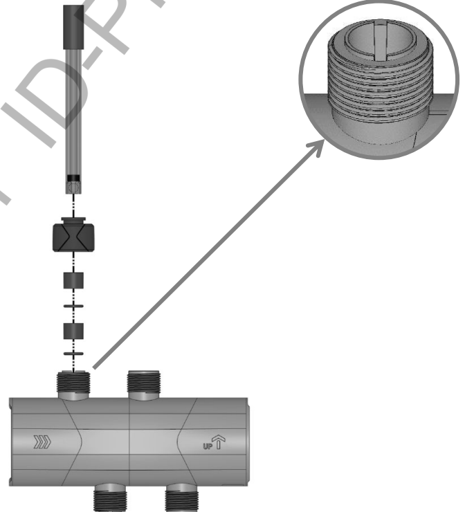
Sonde (pH of ORP) met sondehouder
