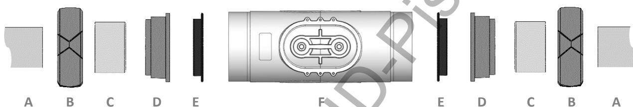
Vista explodida da montagem:
